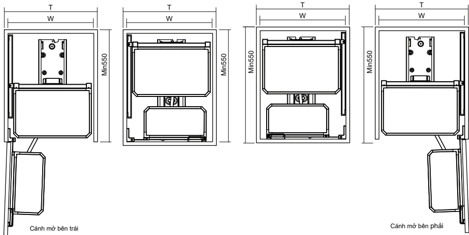
Cánh mở bên trái
