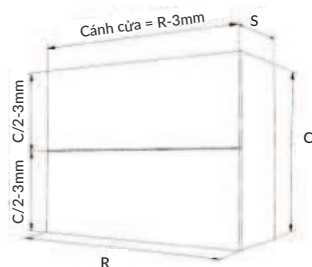
Độ mở cánh cửa lên tối đa
